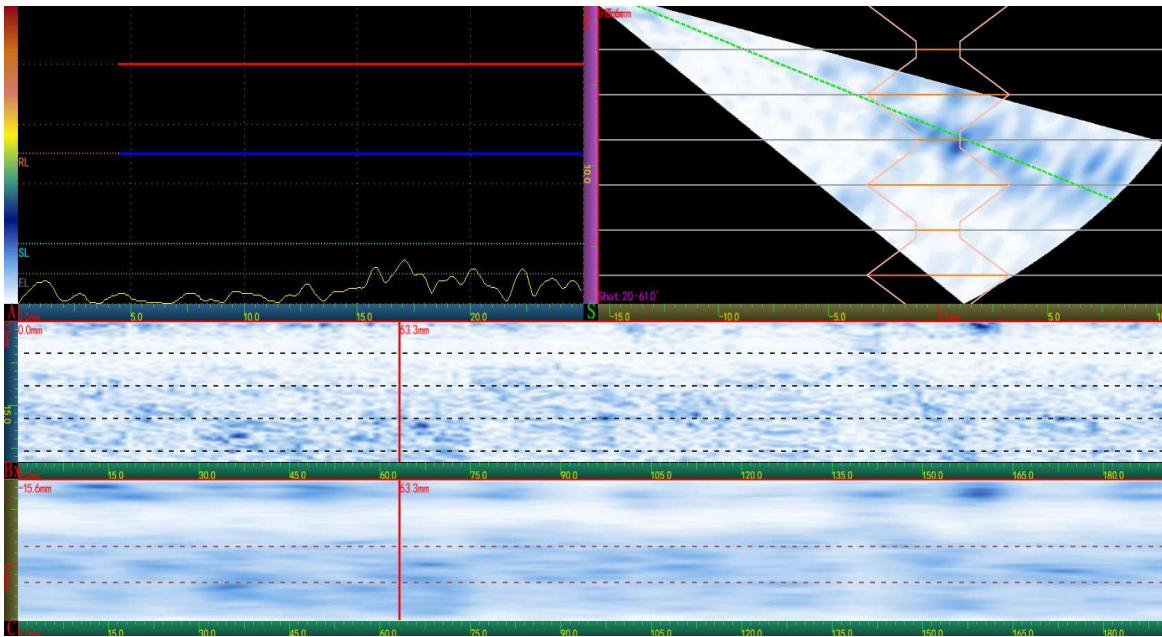
SPOOL-010 JUNTA-042
